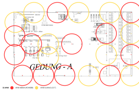
Gambar 3.3. 2 Perencanaan Ulang Layout APAR Gedung A
