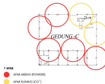
Gambar 3.3. 4 Perencanaan Ulang Layout APAR Gedung B
